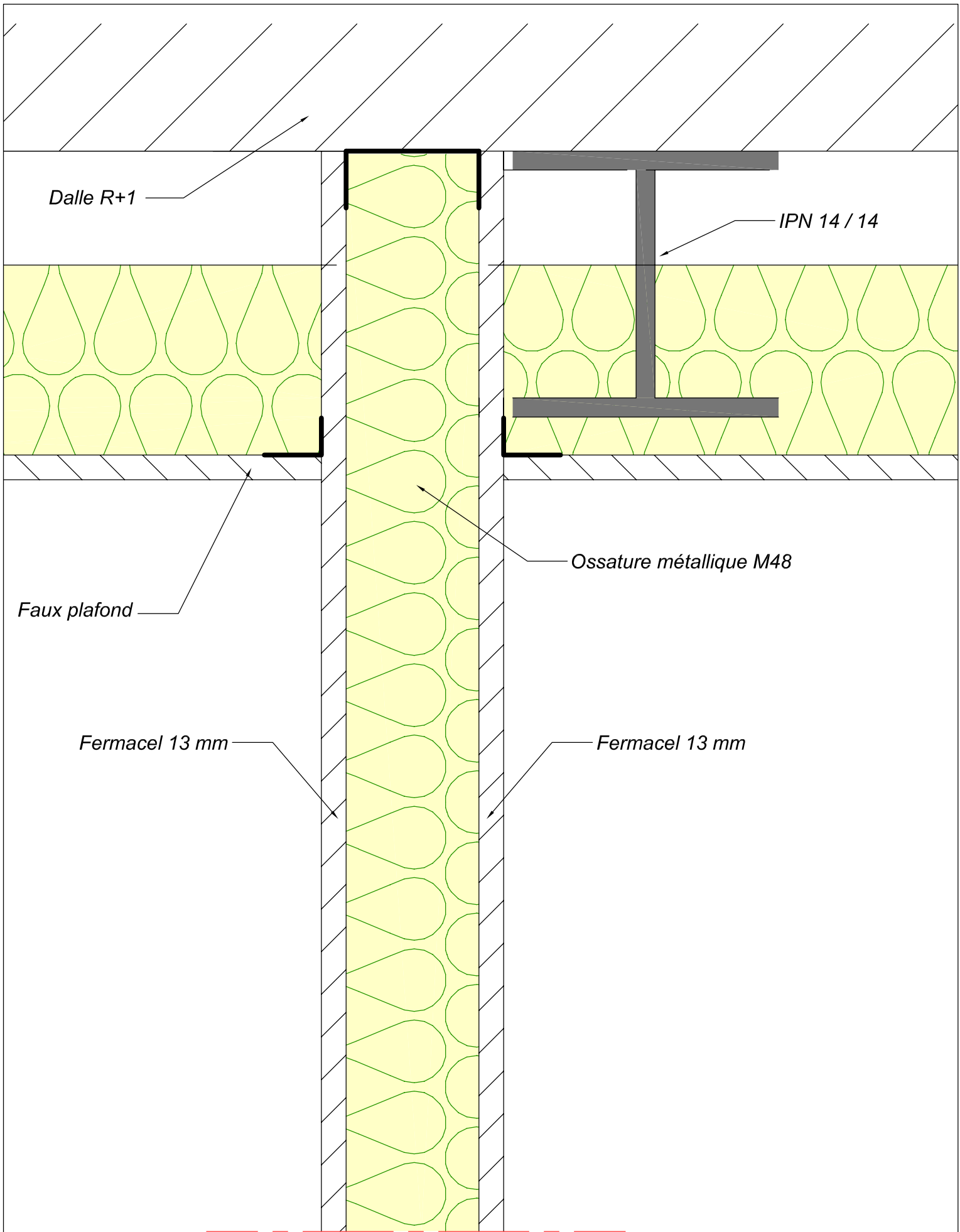
Détail mur n° 2
