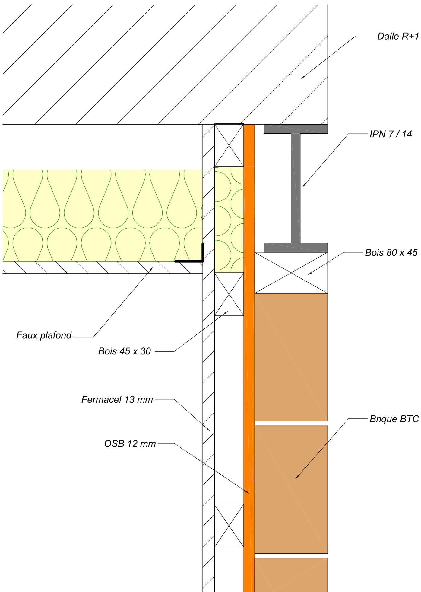
Détail mur n° 3
